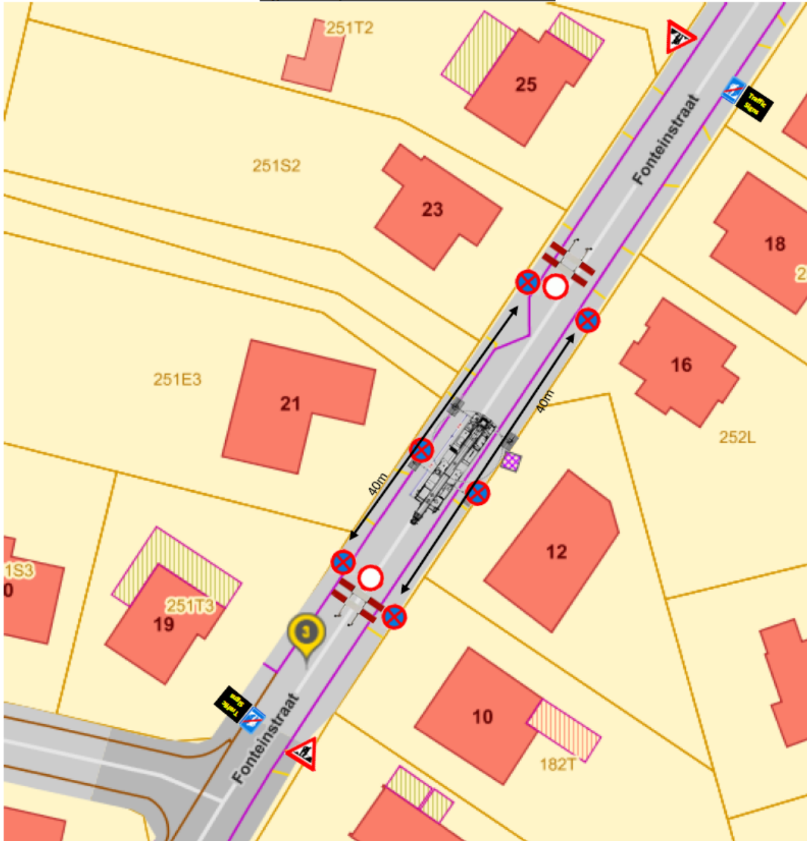
Signalisatieplan – Lubbeek – Fonteinstraat
