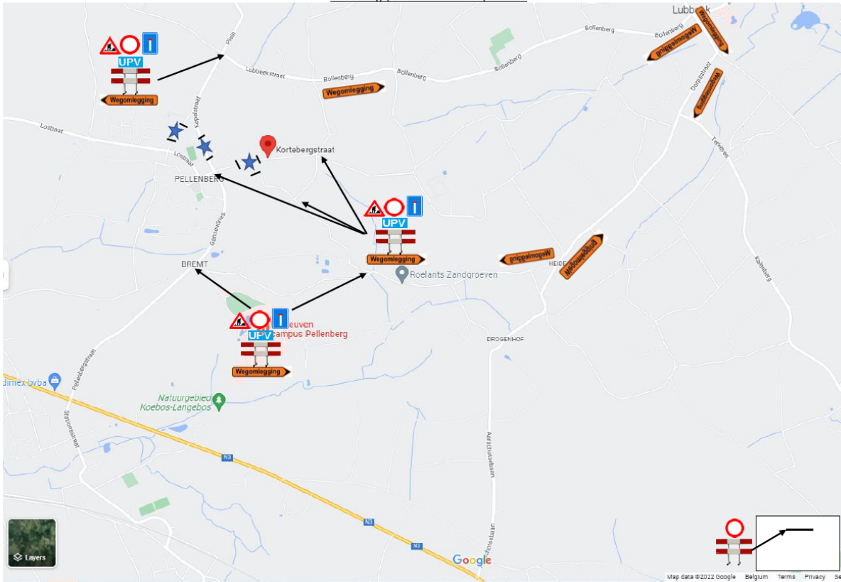
Omlleidingsplan – Lubbeek - Kapelstraat
